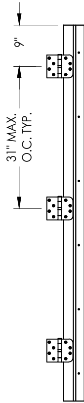
HINGE JAMB
